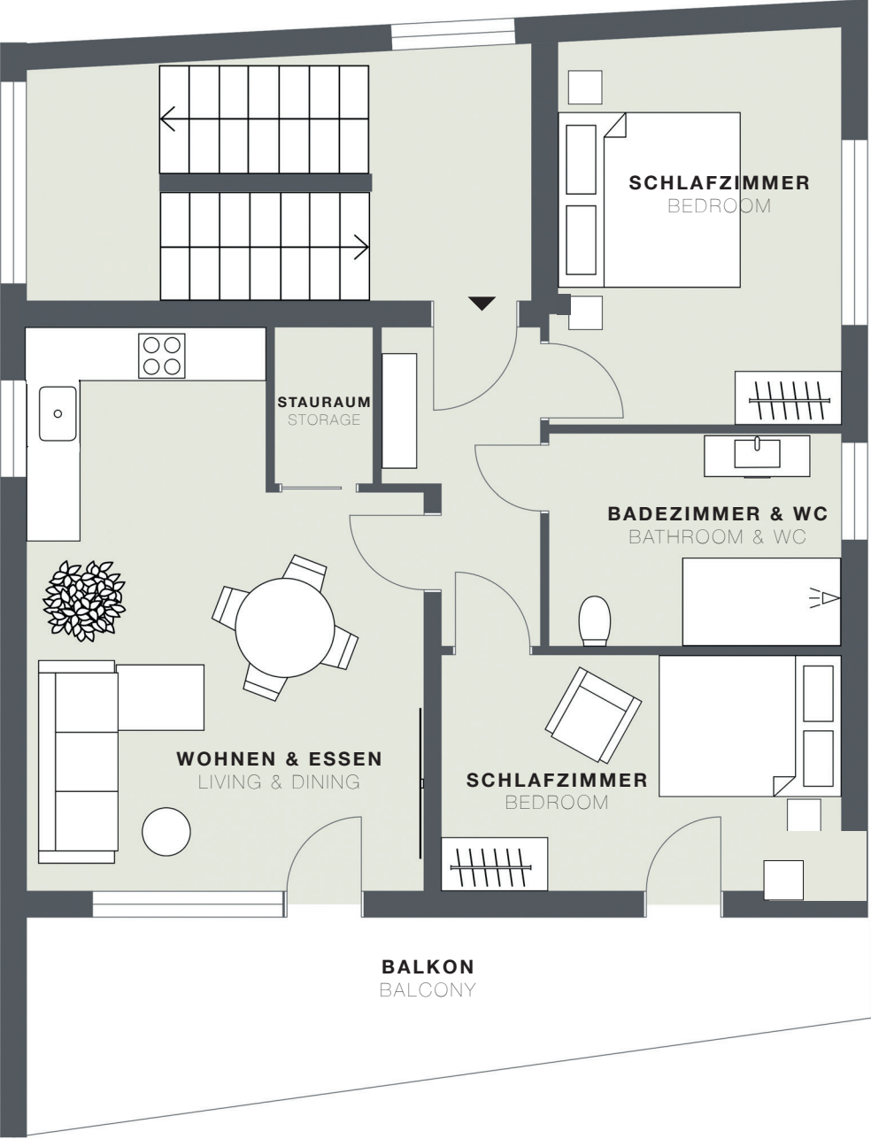
OBERGESCHOSS / UPPER FLOOR
